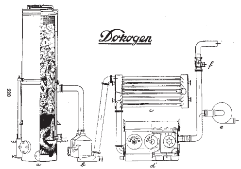
Holzvergassgenerator DOKOGEN – 1938
